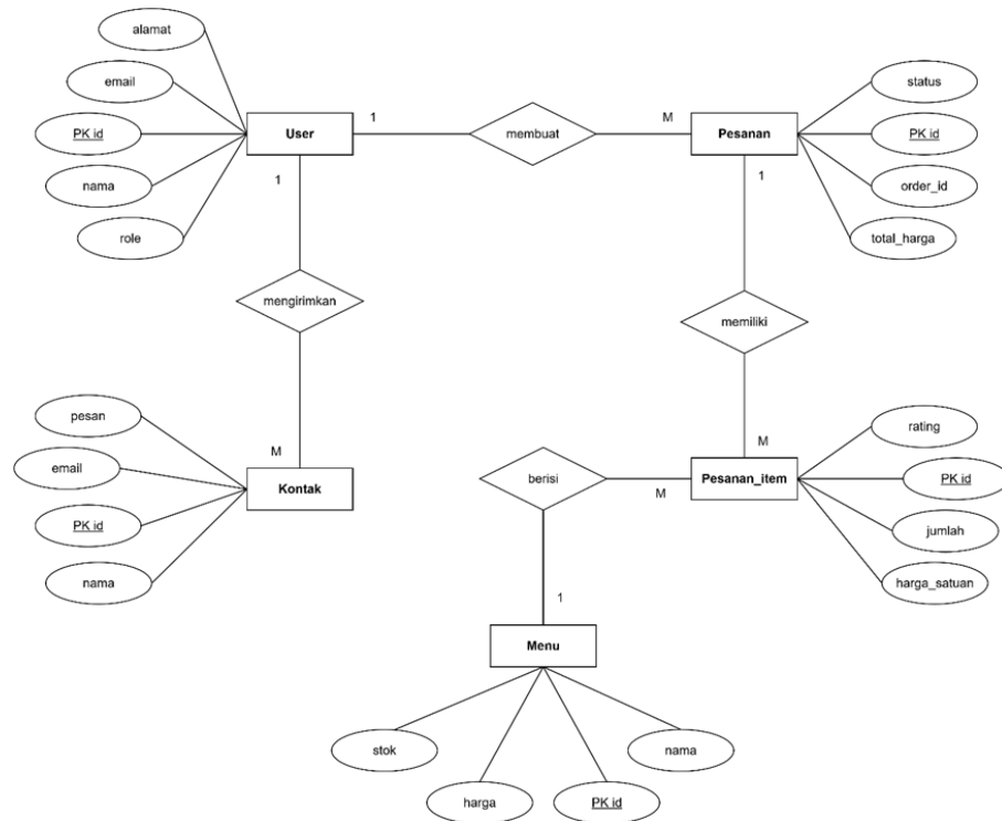
Gambar 3. Diagram Er
