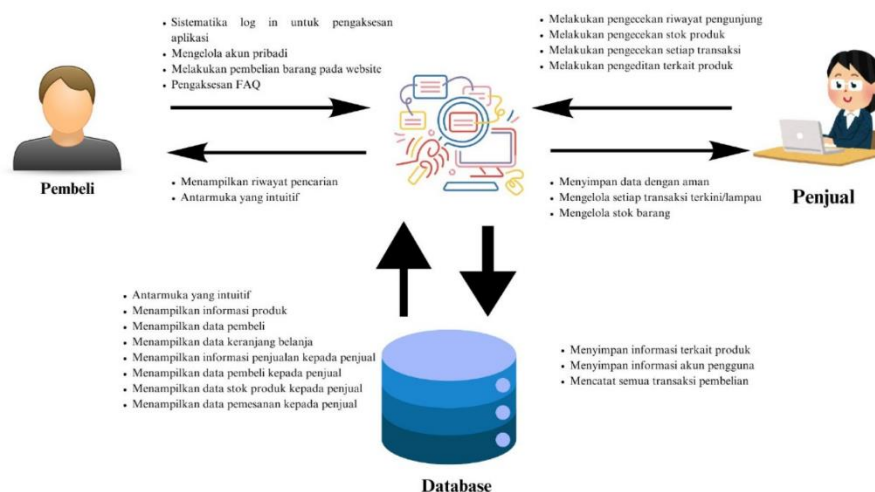
Gambar 1. Deskripsi Umum
